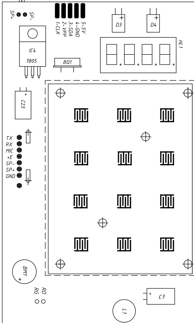
Плата БВД-342R Сборочный чертеж
