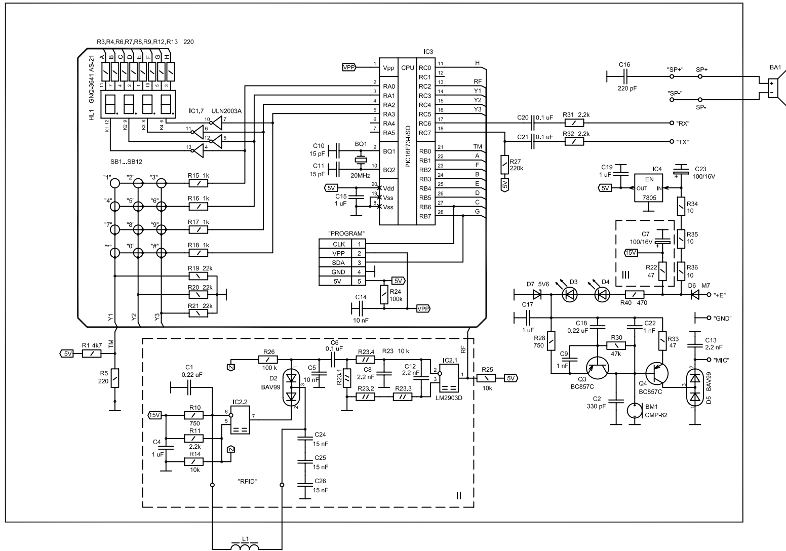
Блок вызова БВД-342 Схема электрическая принципиальная
