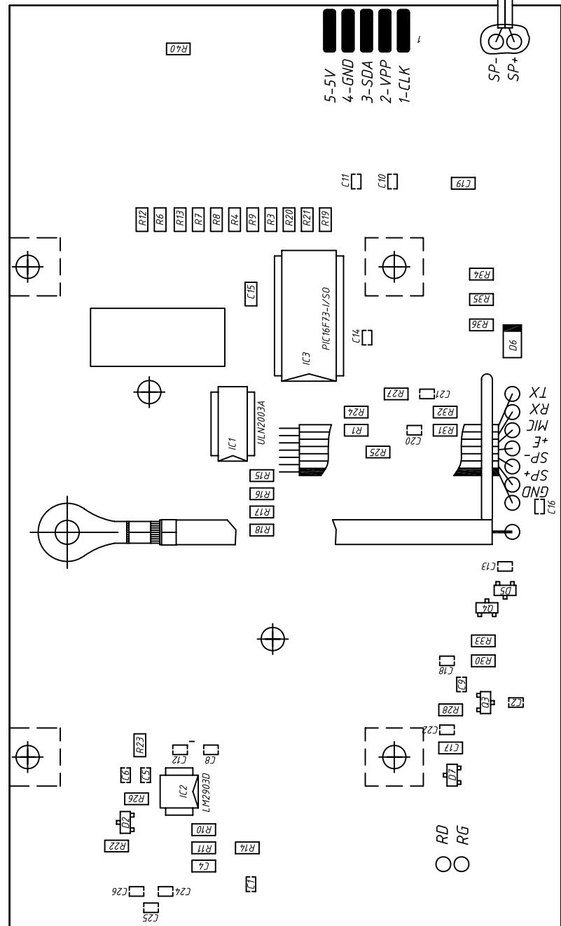
Плата БВД-342R Сборочный чертеж
