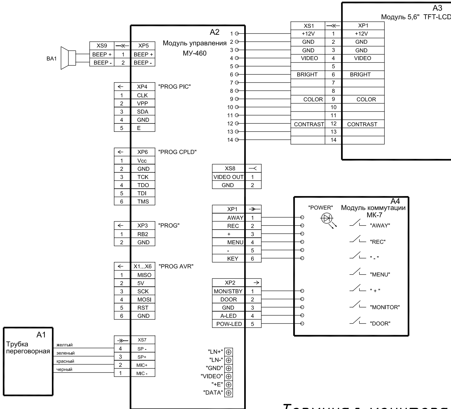
Терминал монитора VIZIT-MT460CM Схема соединений
